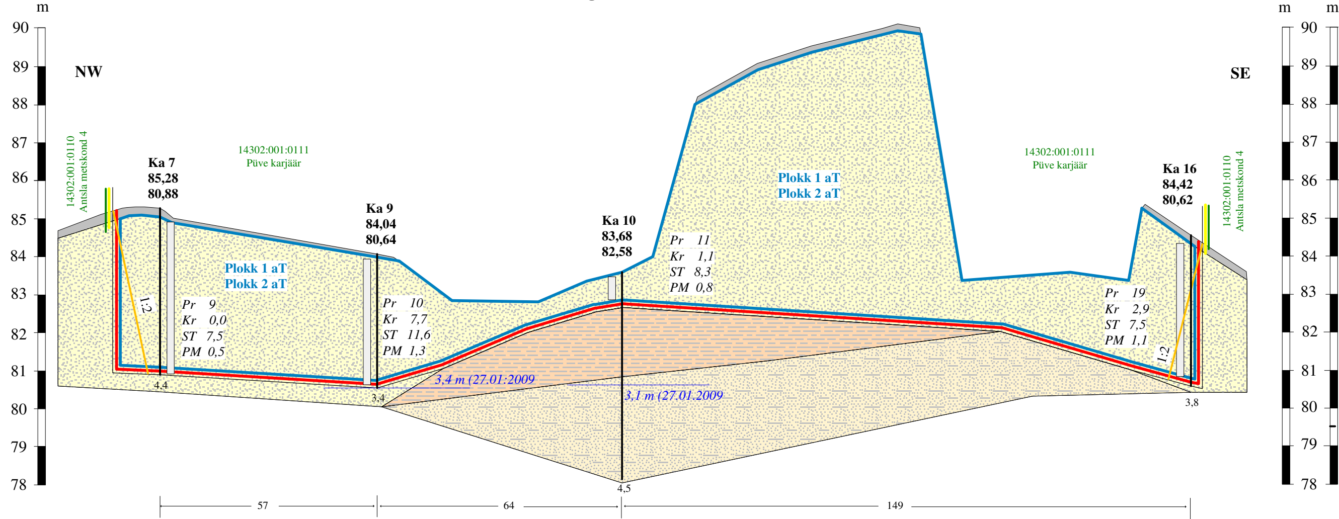
Läbilõige A-B
